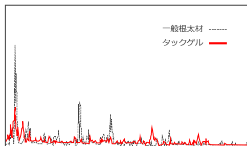
2階からハンマーで叩いた時の衝撃値
